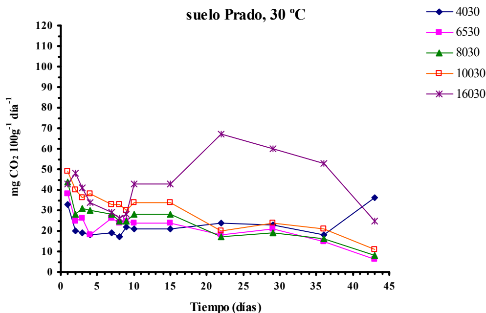
Figura 5.17.- Evolución a lo largo de la incubación a 30 °C de la velocidad de respiración (mg CO 2 emitido 100 g -1 día -1 ) del suelo Prado con diferentes niveles de humedad.
