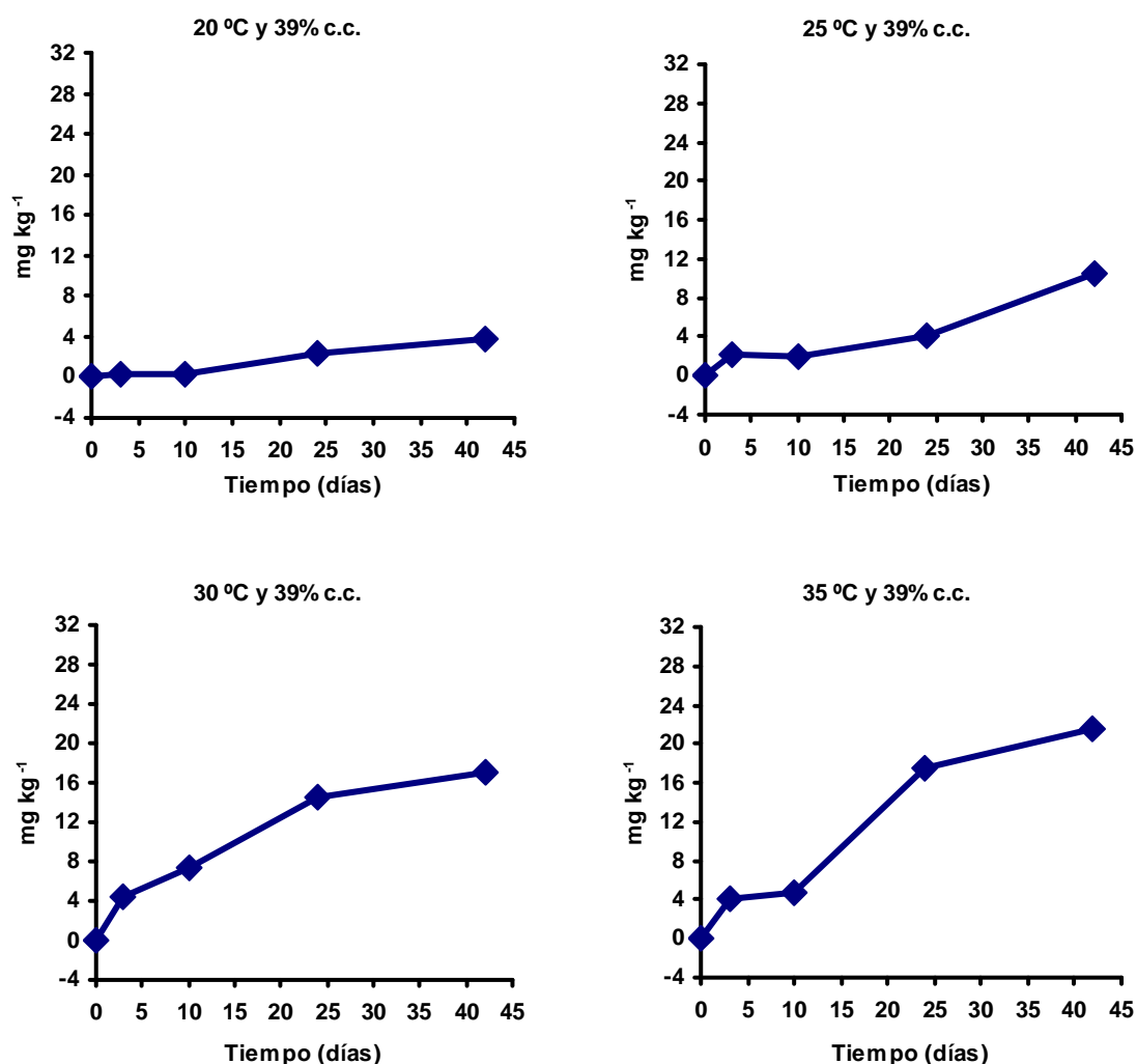
Figura 5.101.- Suelo Robledal: serie de gráficas correspondientes a los datos de mineralización neta acumulada de las formas de Nitrógeno total inorgánico ( N_{min} - N_{tinorg} ) obtenidos para los tiempos control (3, 10, 24 y 42 días) durante las incubaciones realizadas con el suelo humectado al 39% c.c. sometido a las diferentes temperaturas de ensayo.
