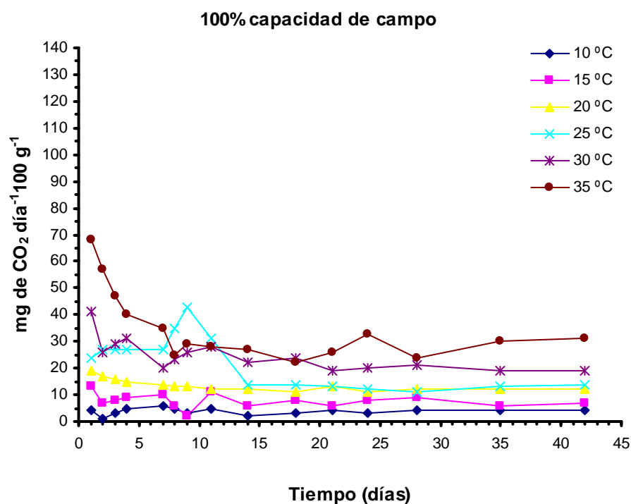
Figura 5.79.- Suelo Robledal: evolución de la velocidad de respiración a 100% c.c. para las distintas temperaturas de incubación.
