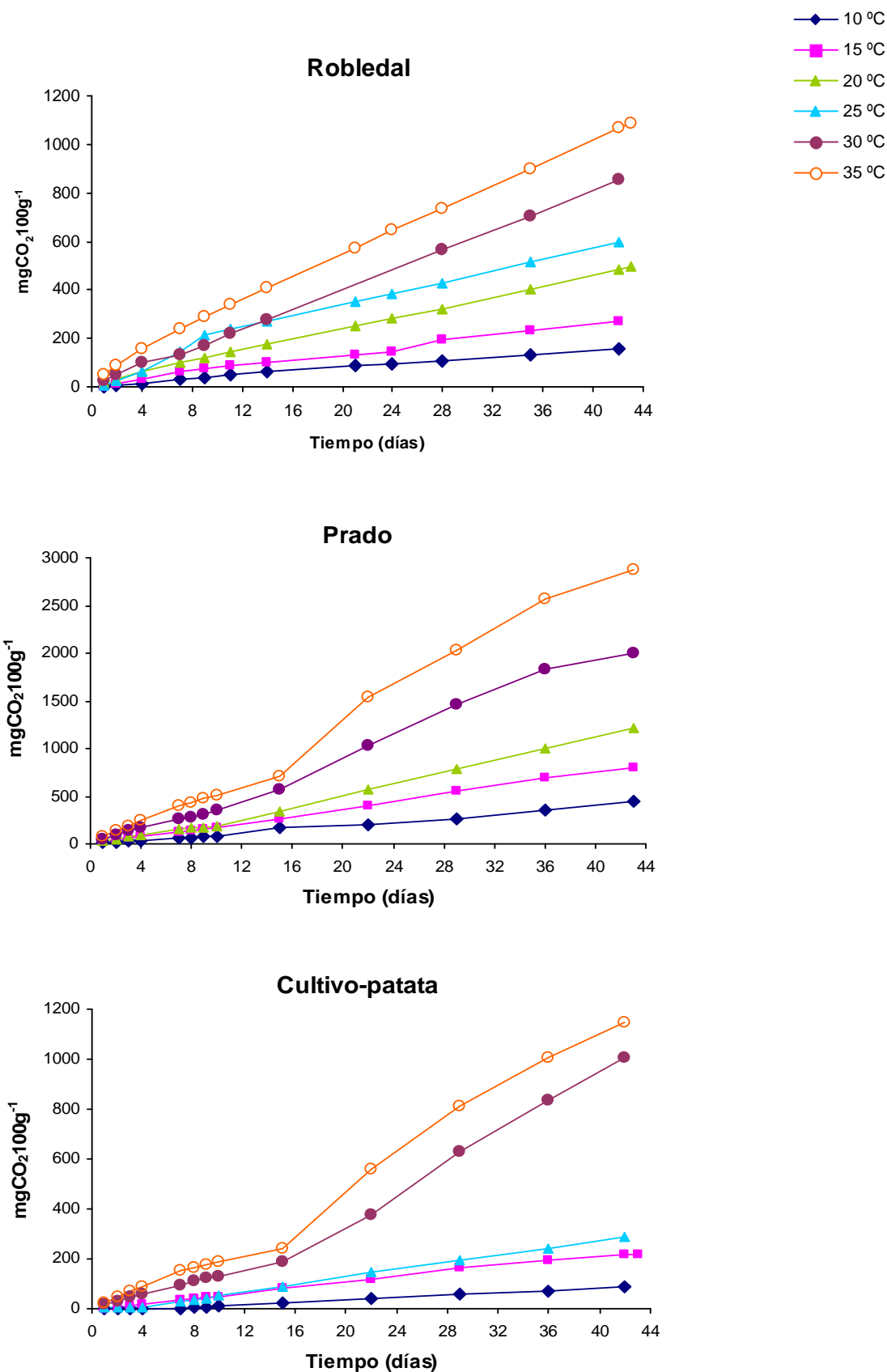
Figura 6.16.- Emisiones de CO 2 absolutas de los tres suelos a lo largo del período de incubación, obtenidas para cada una de las temperaturas en las muestras humectadas al 160% de humedad de la capacidad de campo.
