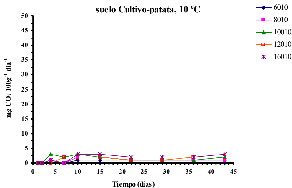
Figura 5.25.- Evolución a lo largo de la incubación a 10 °C de la velocidad de respiración ( \text{mg CO}_2 emitido 100 \text{ g}^{-1} \text{ día}^{-1} ) del suelo Cultivo-patata con diferentes niveles de humedad.
