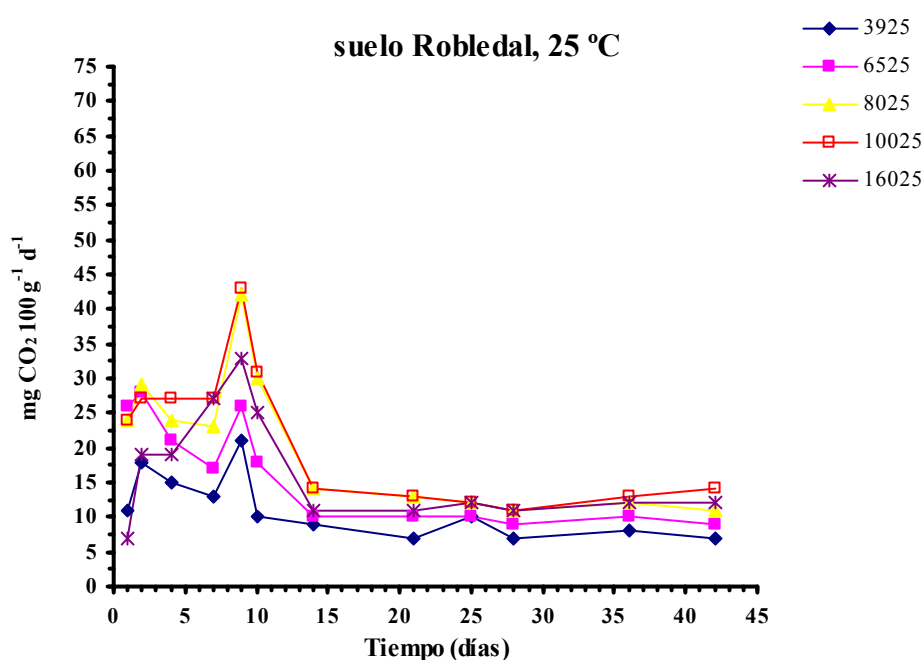
Figura 5.4.- Evolución a lo largo de la incubación a 25 °C de la velocidad de respiración ( \text{mg CO}_2 emitido 100 \text{ g}^{-1} \text{ día}^{-1} ) del suelo Robledal con diferentes niveles de humedad.
