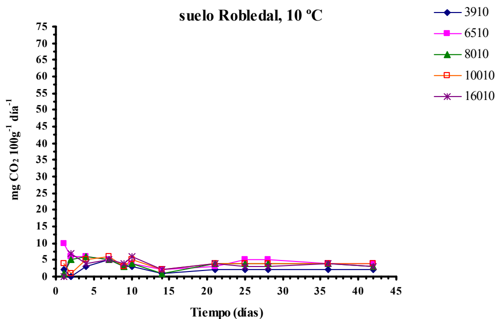
Figura 5.1 .- Evolución a lo largo de la incubación a 10 °C de la velocidad de respiración ( \text{mg CO}_2 \text{ g}^{-1} \text{ día}^{-1} ) del suelo Robledal con diferentes niveles de humedad.
