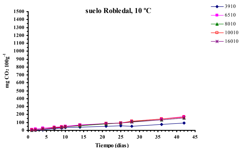
Figura 5.7.- Emisión de CO 2 acumulada (mg de CO 2 100 g -1 ) obtenida a lo largo de la incubación para el suelo Robledal incubado a 10 °C y con diferentes niveles de humedad.
