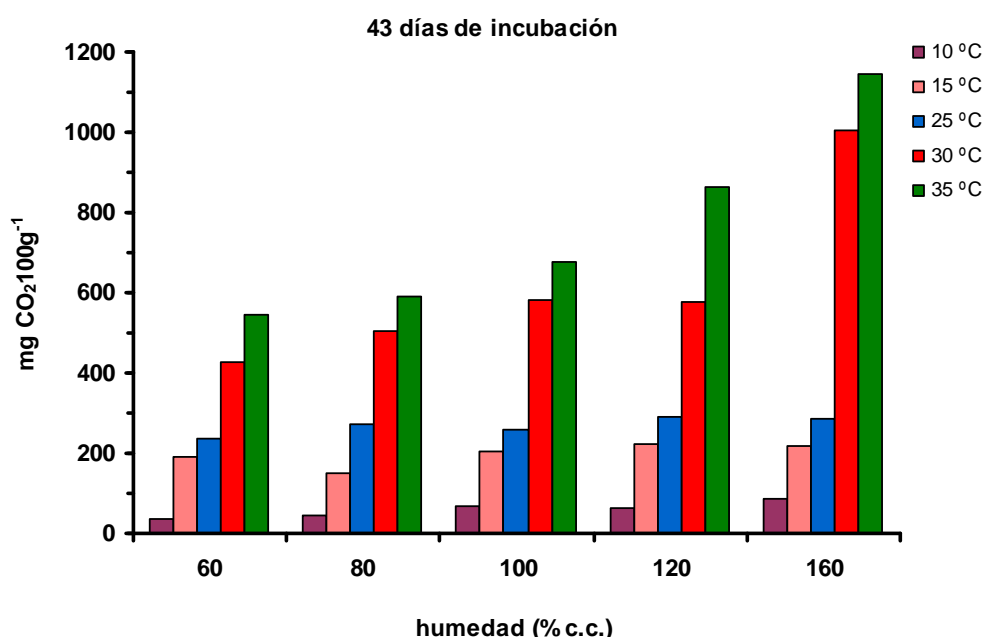
Figura 5.44.- Suelo Cultivo-patata: influencia de la humedad sobre la emisión acumulada de CO 2 a los 15 días de incubación, a las distintas temperaturas.
